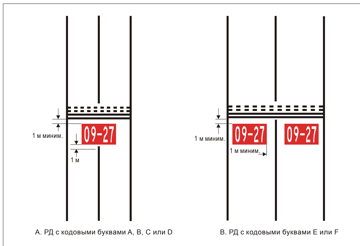
Рис. 5-10. Маркировка, содержащая обязательные для исполнения инструкции
