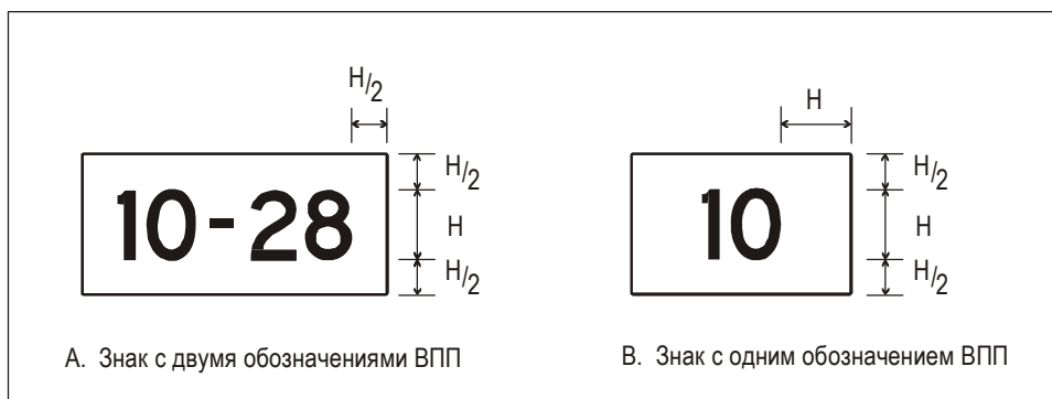
Рис. А4-3. Размеры знака
