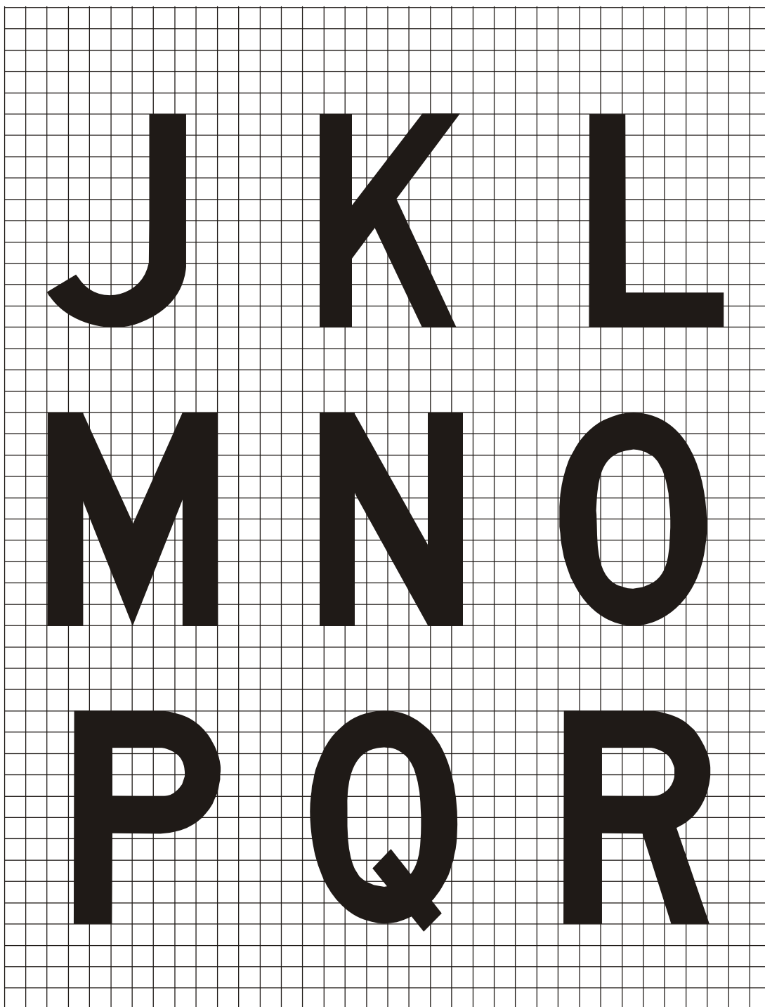
Рис. А4-2. Форма знаков (продолж.)
