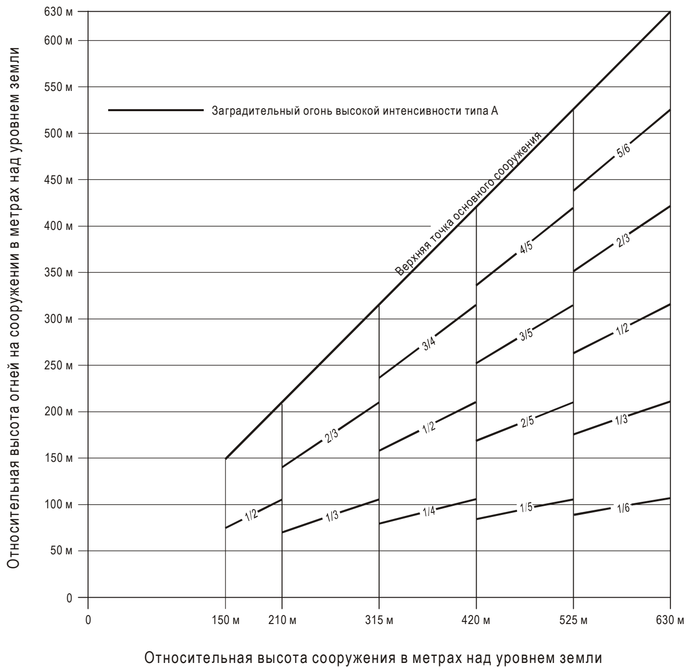
Рис. А6-6. Система светоограждения препятствий с белыми проблесковыми огнями высокой интенсивности типа А
