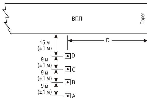
Типовой фланговый горизонт PAPI
