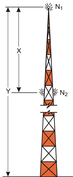
Рис. 6-2. Примеры маркировки и светового ограждения высоких сооружений
