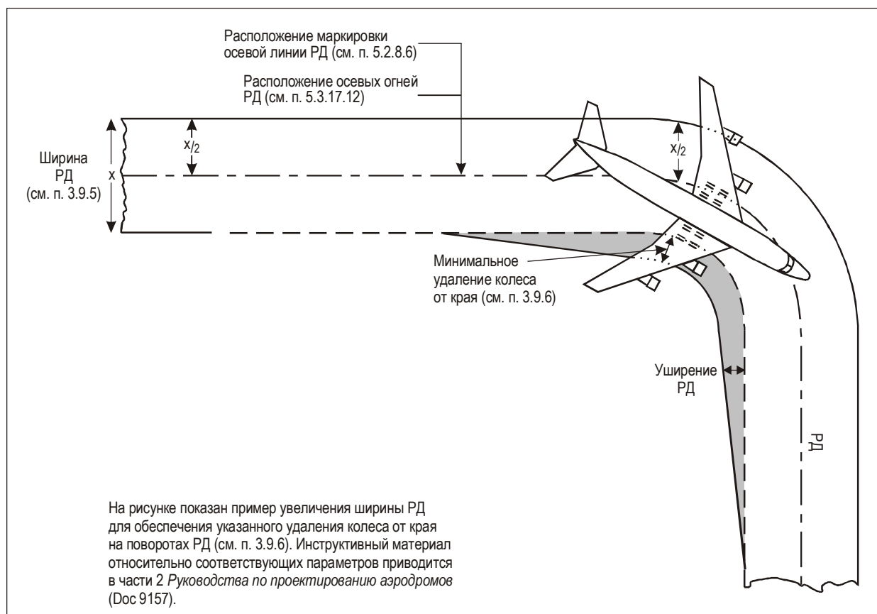
Рис. 3-2. Поворот РД
